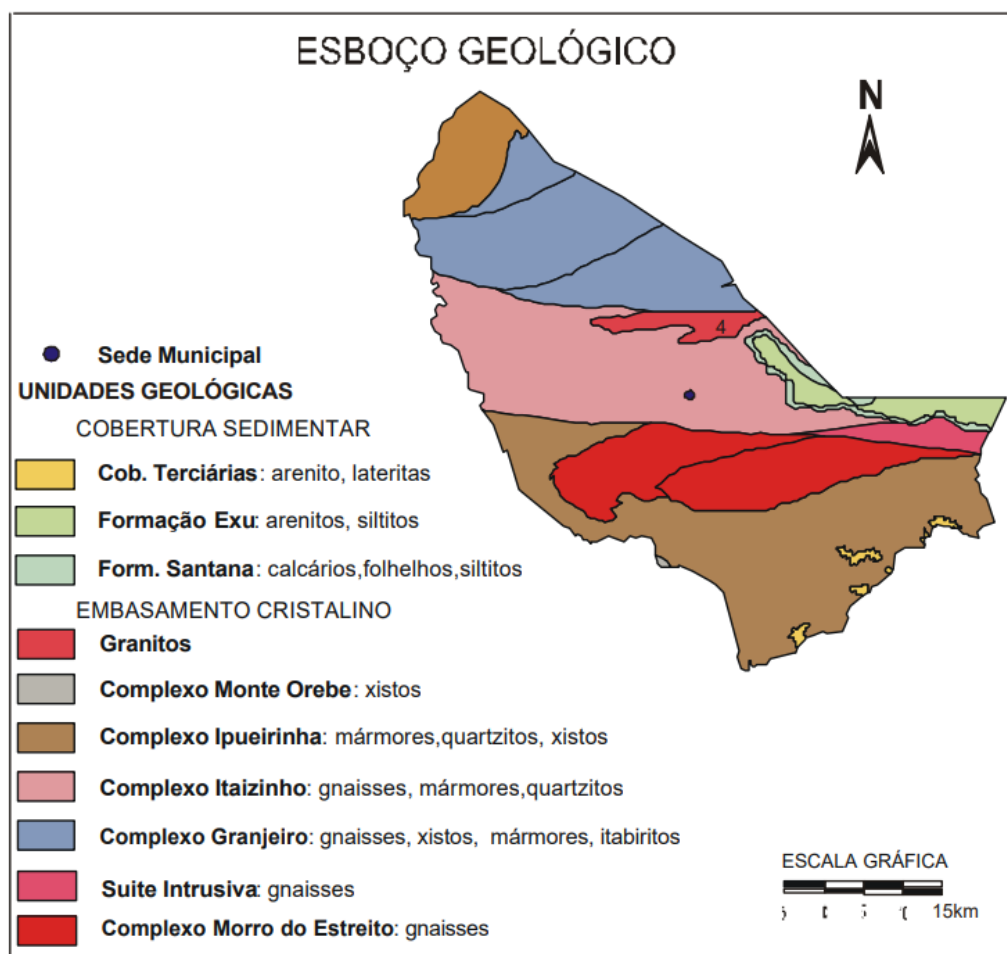
Esboço Geológico do município.
